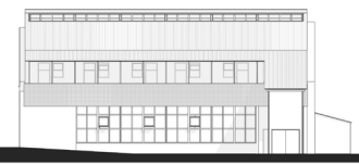
Pohled severní - 1:200
