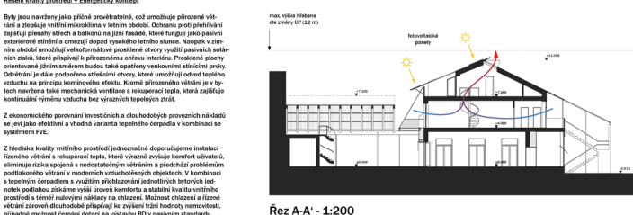
Řez A-A' - 1:200
