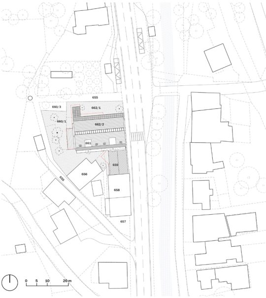
Situace celková - 1:500
