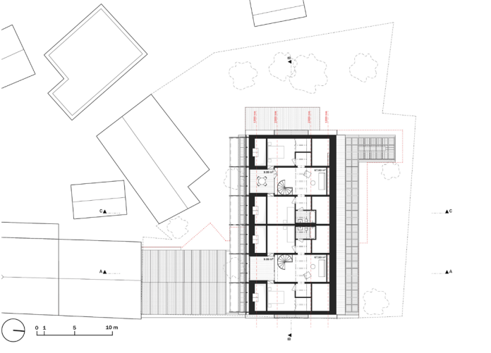
Půdorys podkrovní - 1:200
