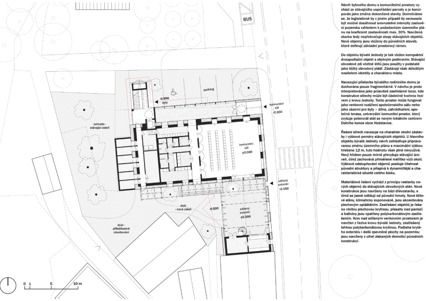
Situace koordinační - 1:200
