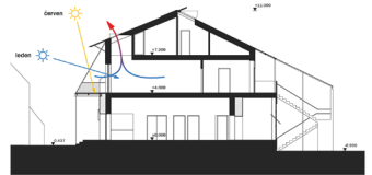
Řez C-C' - 1:200
