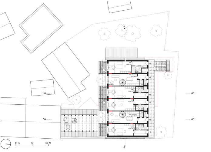
Půdorys 2.NP - 1:200
