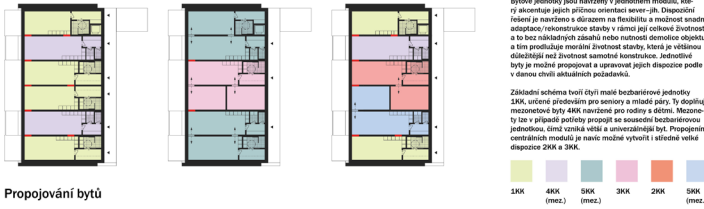
Propojování bytů
