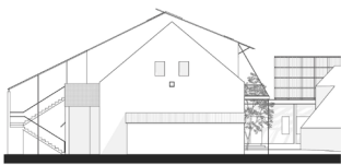
Pohled západní - 1:200
