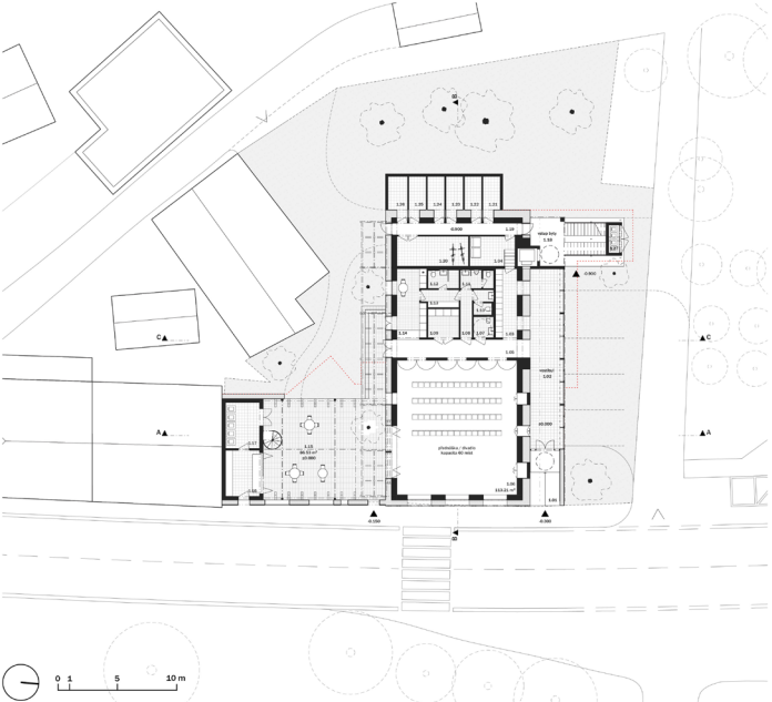
Půdorys 1.NP - 1:200
